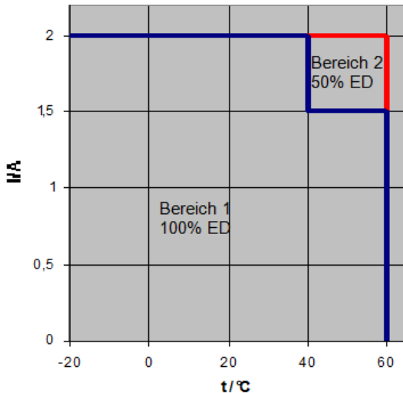
Abbildung 1: Einschaltdauer in Abhängigkeit des Laststroms und Umgebungstemperatur
